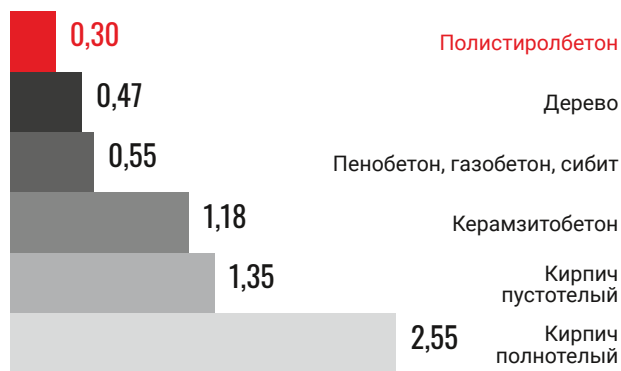
Толщина стены при одинаковой теплопроводности, метров
